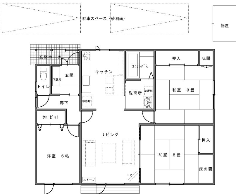
【緑酔庵図面】
